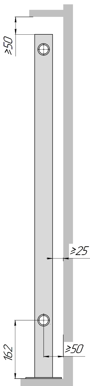
QUADRUN NEO 50 V FF (вид сбоку)
