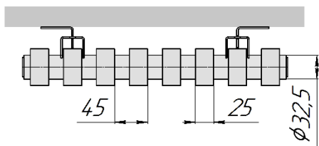
QUADRUN NEO 50 V (вид сверху)
