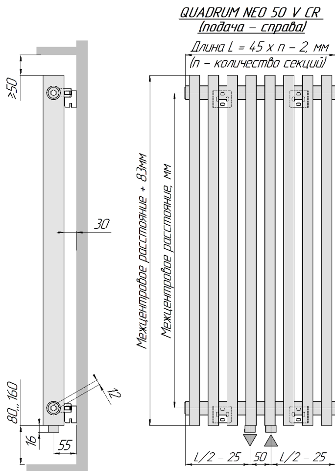
QUADRUN NEO 50 V CR (вид сбоку, кронштейны КС 14)
