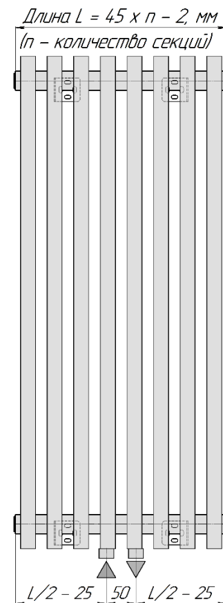
QUADRUN NEO 50 V CL (подача – слева)
