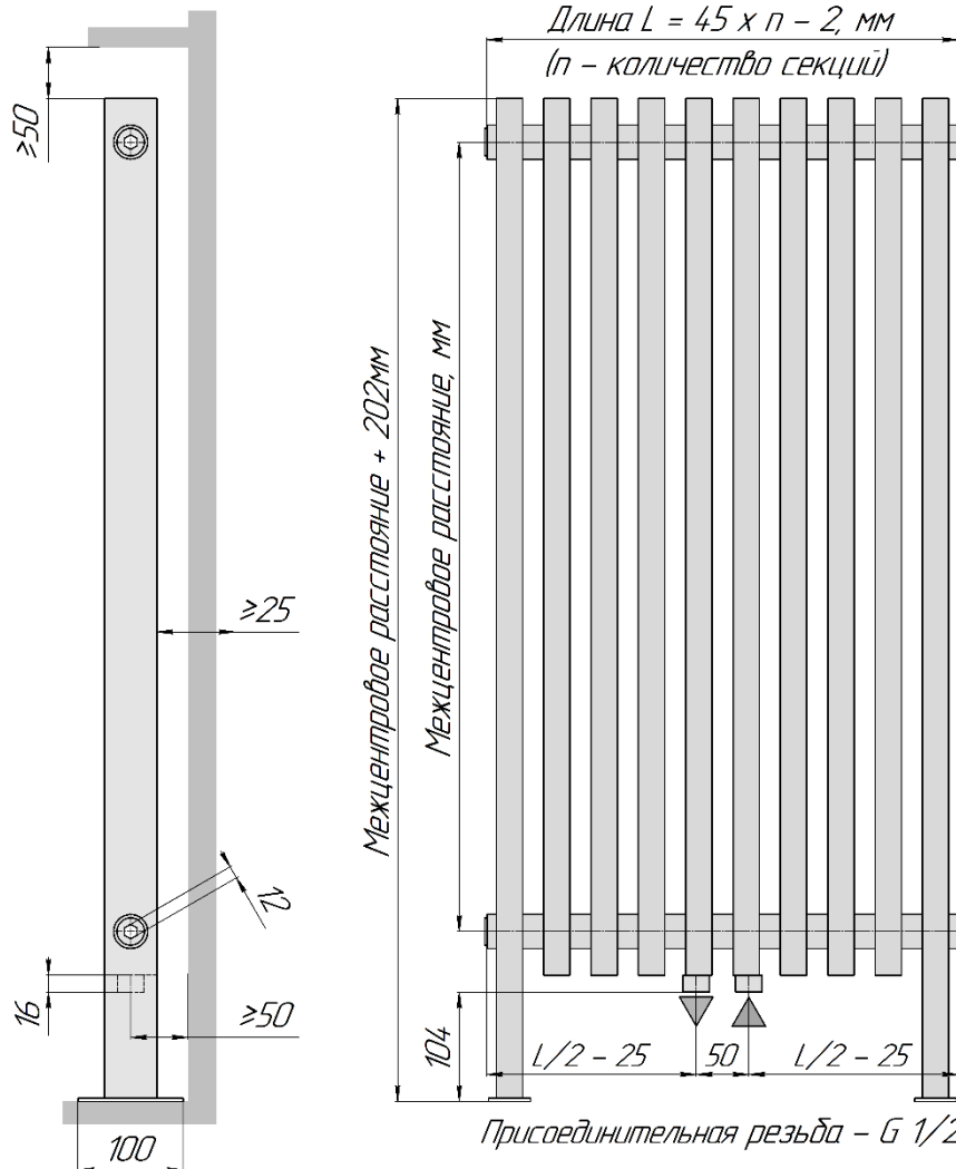
QUADRUN NEO 50 V CR FF (вид сбоку)
