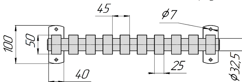
QUADRUN NEO 50 V FF (вид сверху)
