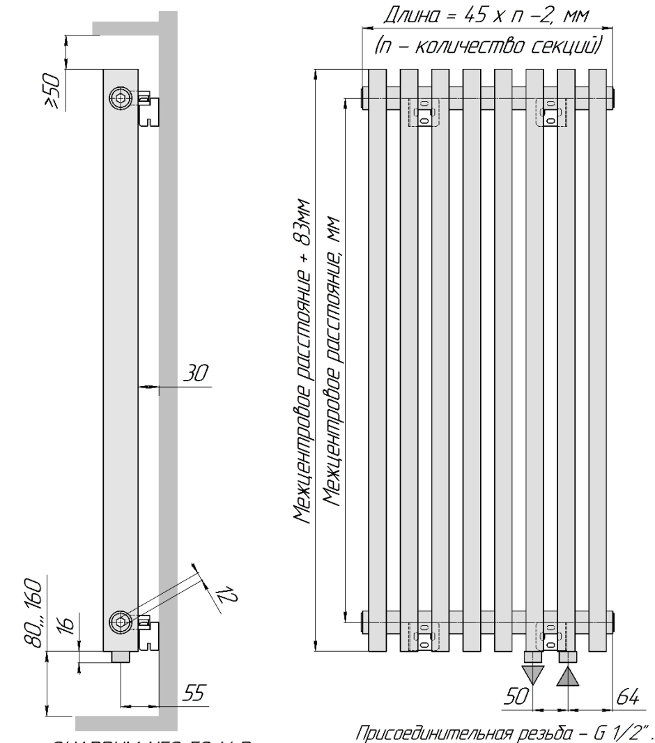
QUADRUN NEO 50 V R (вид сбоку, кронштейны КС 14)
