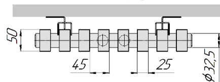
QUADRUN NEO 50 V CR (вид сверху)
