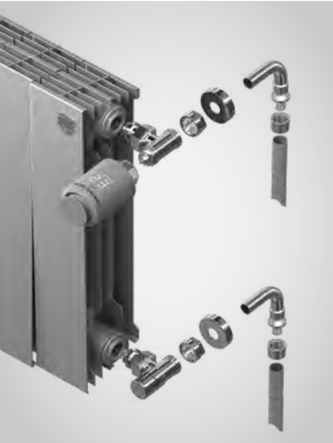
Набор термостатический Design PRO под трубку Ø15 мм, угловой, хром
